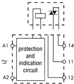
Schema di collegamento modelli in AC Wiring diagram AC models
