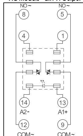
Modelli in AC - Uscita 2x1 A AC Models - 2x1 A Output
