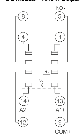
Modelli in DC - Uscita 1x10 A DC Models - 1x10 A Output
