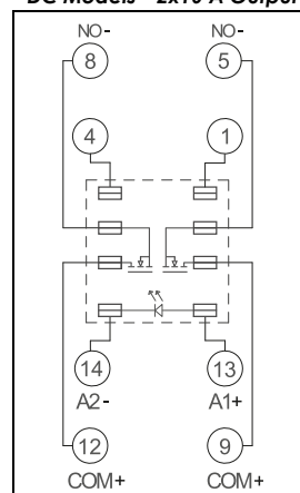
Modelli in DC - Uscita 2x10 A DC Models - 2x10 A Output
