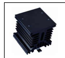
HS3-120: 125 x 120 x 141 (h) HS3-120 + SSR: 125 x 120 x 179 (h)
